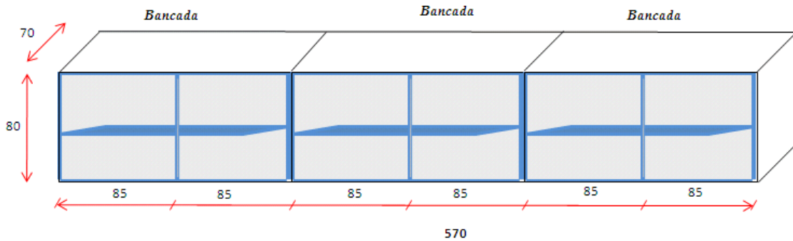
Figura 4 - Armário de 570 x 80 x 70 (LxAxP), com uma prateleira e duas portas de correr. (Extração de solos)
