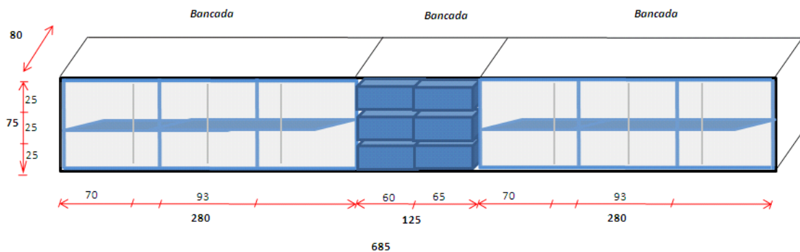
Figura 8 - Armário de 685 x 75 x 80 (LxAxP), com uma prateleira, seis portas de correr e seis gavetas, para bancada de fundo.
