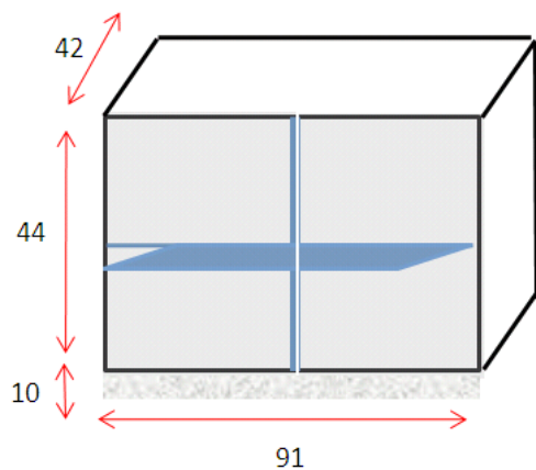
Figura 2 - armário inferior de 70 x 91 x 44 cm (A x L x P), sob a pedra. (lavabo )
