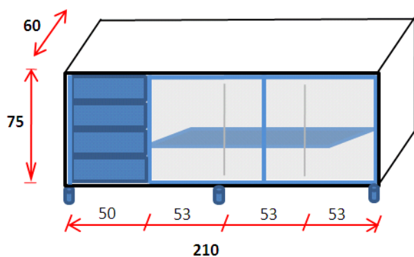
Figura 1 - Um armário inferior de 76 x 210 x 60 cm (A x L x P), com quatro gavetas, três portas e seis pés. (Copa)
