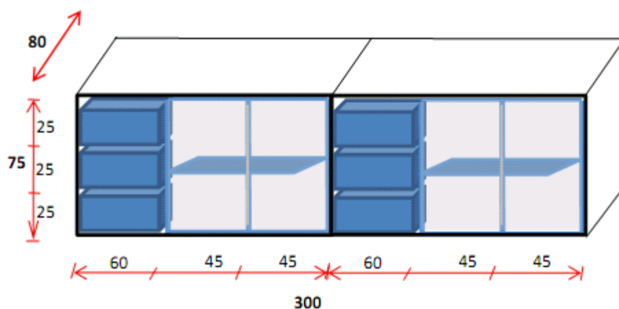
Figura 13 - Armário de 300 x 75 x 80 (LxAxP), com três gavetas, uma prateleira e duas portas de correr, para balanças. (Lab. Analítica)
