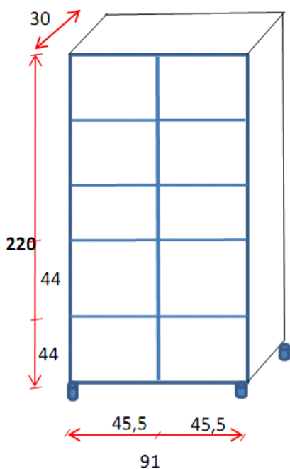
Figura 3 - Armário de 220 x 91 x 30 cm (A x L x P). Lavado
