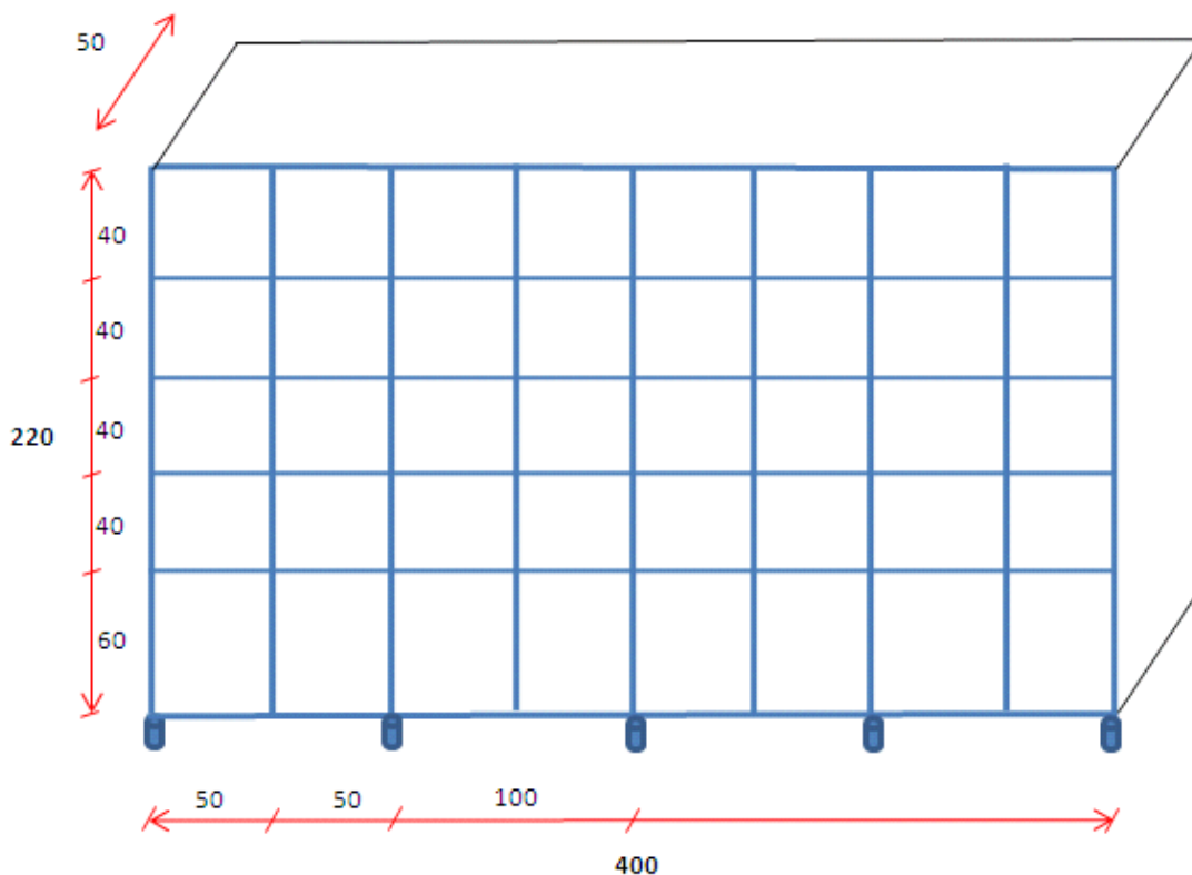
Figura 14 - Armário de 400 x 220 x 50 (LxAxP), com pé, sem portas, com prateleiras para 40 divisões de 60x40 e 40x40, para depósito de reagentes. (Almoxarifado)
