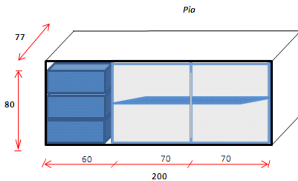
Figura 9 – Armário de 200 x 80 x 77 (LxAxP), com três gavetas, uma prateleira e duas portas de correr, para pia. (lab Solos)
