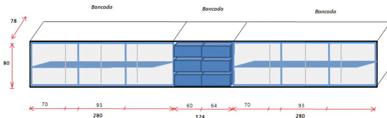
Figura 11 - Armário de 684 x 80 x 78 (LxAxP), com uma prateleira, seis portas de correr e seis gavetas, para bancada de fundo. (Lab. Analítica)
