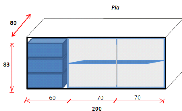
Figura 12 - Armário de 200 x 83 x 80 (LxAxP), com três gavetas, uma prateleira e duas portas de correr, para pia (Lab. Analítica)
