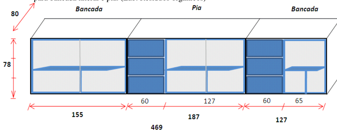
Figura 18 - Armário de 469 x 78 x 80 (LxAxP), com uma prateleira, cinco portas de correr e seis gavetas, para bancada e pia. (Lab. física de solo)
