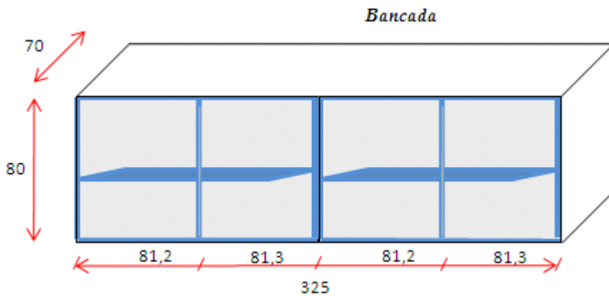
Figura 5 - Armário de 325 x 80 x 70 (LxAxP), com uma prateleira e duas portas de correr. (Extração de solos)
