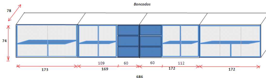
Figura 17 - Armário de 686 x 74 x 78 (LxAxP), com uma prateleira, nove portas de correr e seis gavetas, para bancada lateral e pia. (Lab. Resíduos orgânicos)
