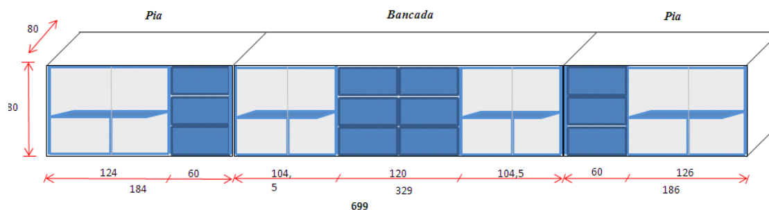
Figura 19 - Armário de 699 x 80 x 80 (LxAxP), com uma prateleira, oito portas de correr e nove gavetas, para bancada lateral e pia. (Lab. de Água)
