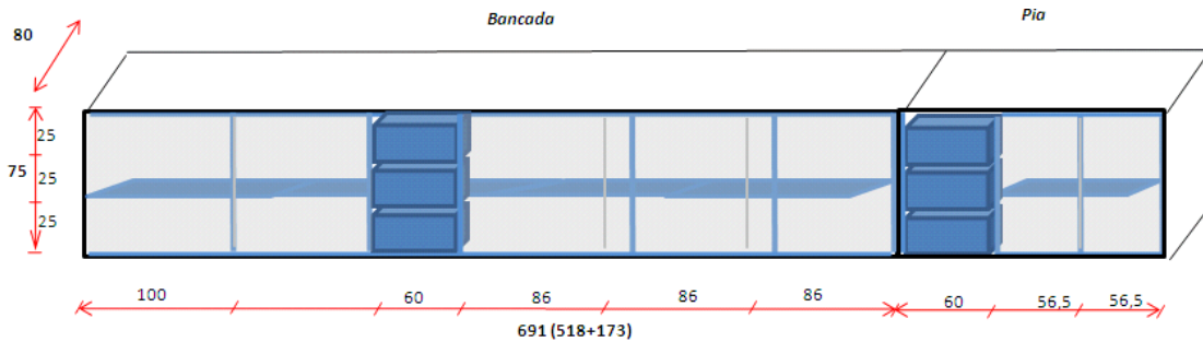
Figura 7 – Um armário de 691 x 75 x 80 (LxAxP), com uma prateleira, sete portas de correr e seis gavetas.
