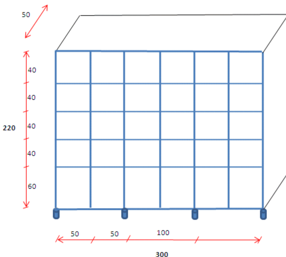
Figura 15 - Armário de 300 x 220 x 50 (LxAxP), com pé, sem portas, com prateleiras para 30 divisões de 60x40 e 40x40, para depósito de reagentes. (Almoxarifado)
