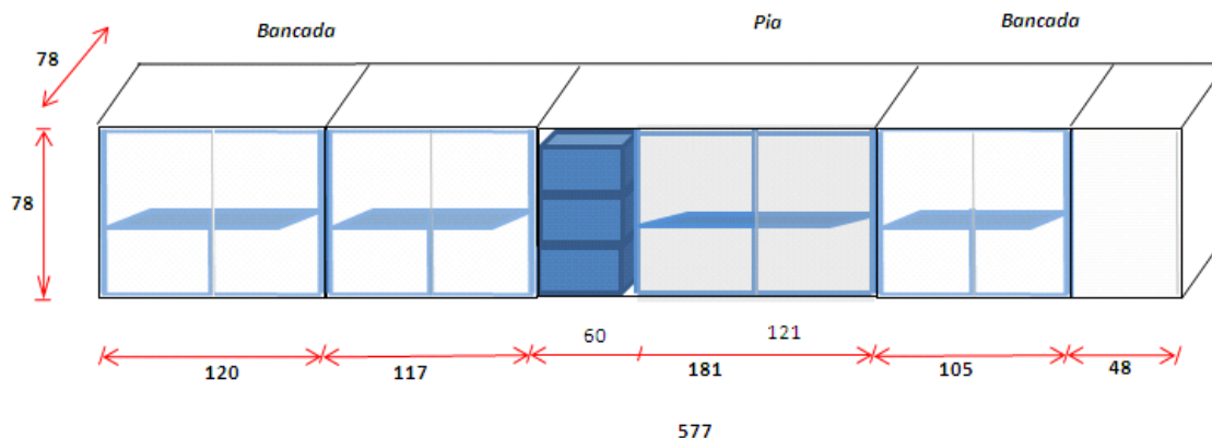
Figura 16 - Armário de 577 x 78 x 78 (LxAxP), com uma prateleira, nove portas de correr e três gavetas, para bancada de fundo e pia (Lab. Resíduos orgânicos)
