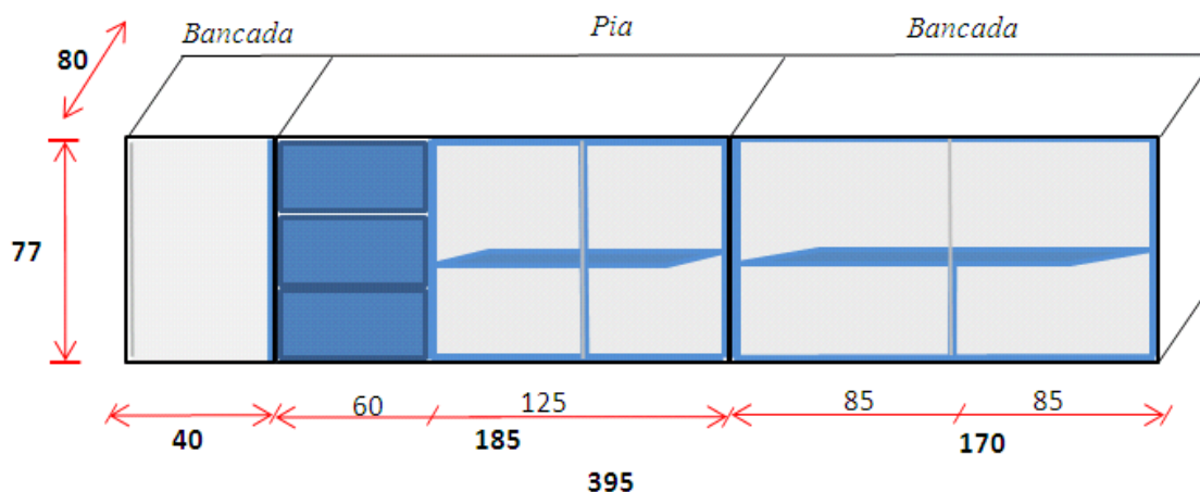
Figura 20 - Armário de 395 x 77 x 80 (LxAxP), com uma prateleira, cinco portas de correr e seis gavetas, para bancada de fundo pia. (Lab. de Água)
